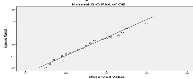
Grafik IV.2 Normal Q-Q plot Kecerdasan Emosional (QE)
