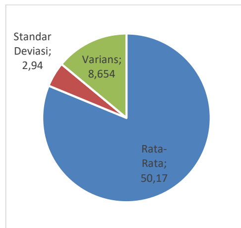
Gambar 4.1 Diagram Kemampuan Awal Peserta Didik
