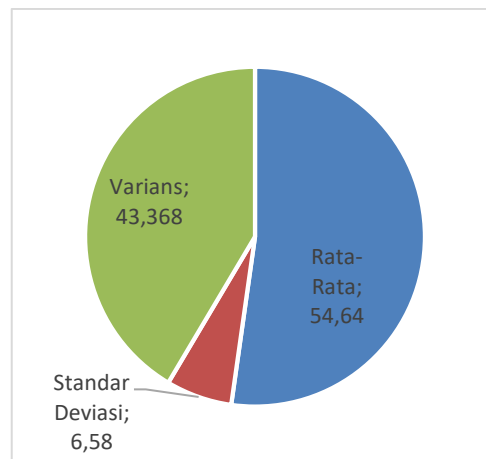
Gambar 4.2 Diagram Kemampuan Akhir Peserta Didik
