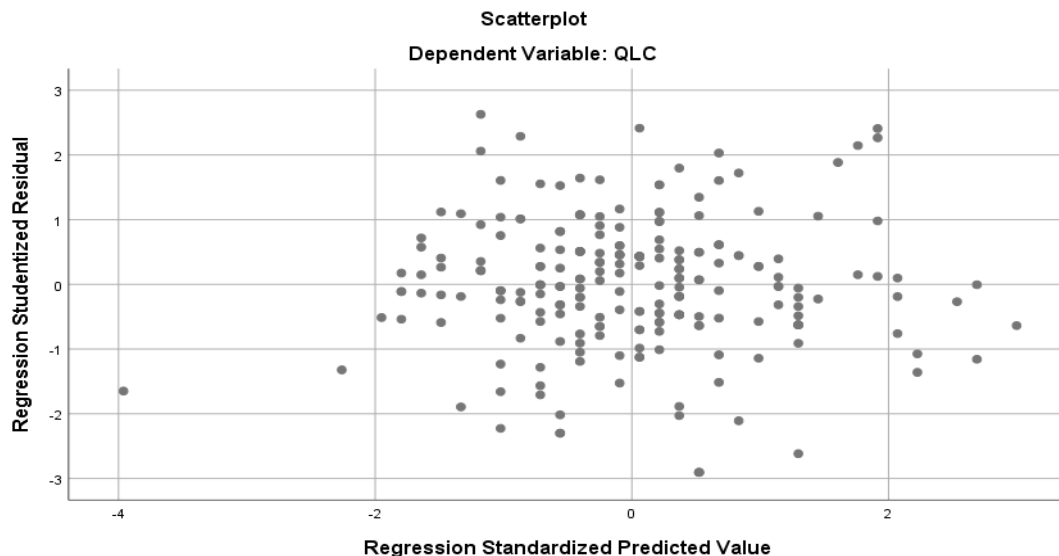
Grafik 4.1 Scatterplot
