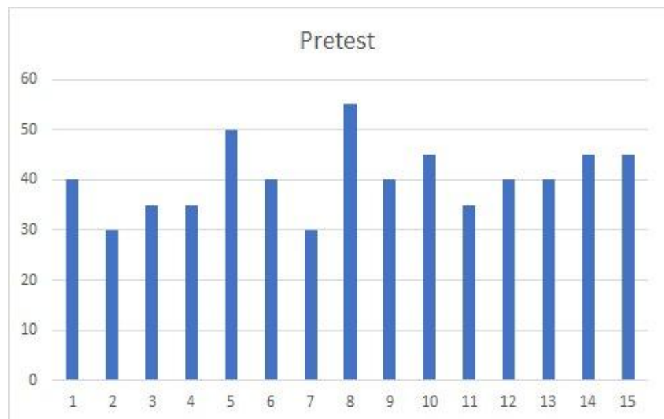
gambar 4.3 Grafik Pretest
