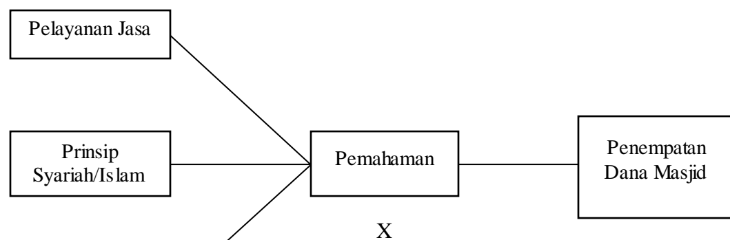
Gambar 1.2: Kerangka Pemikiran
