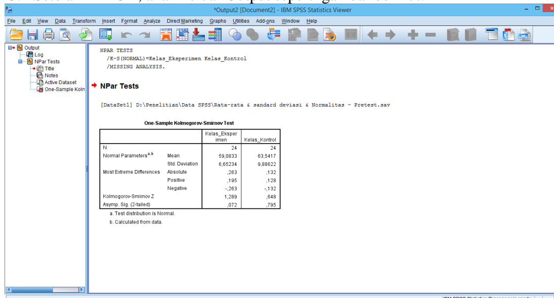
One-Sample Kolmogorov-Smirnov Test
