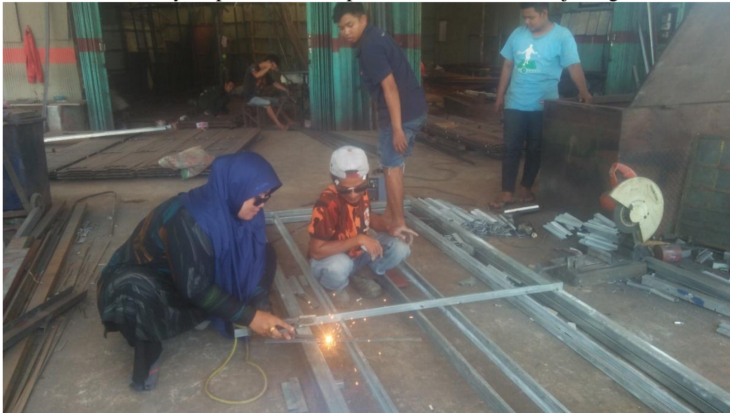
Ibu Asmayani pada saat mempraktikkan cara me-las baja ringan
