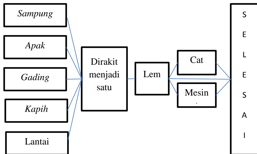
Gambar 4.1 Proses produksi jukung
