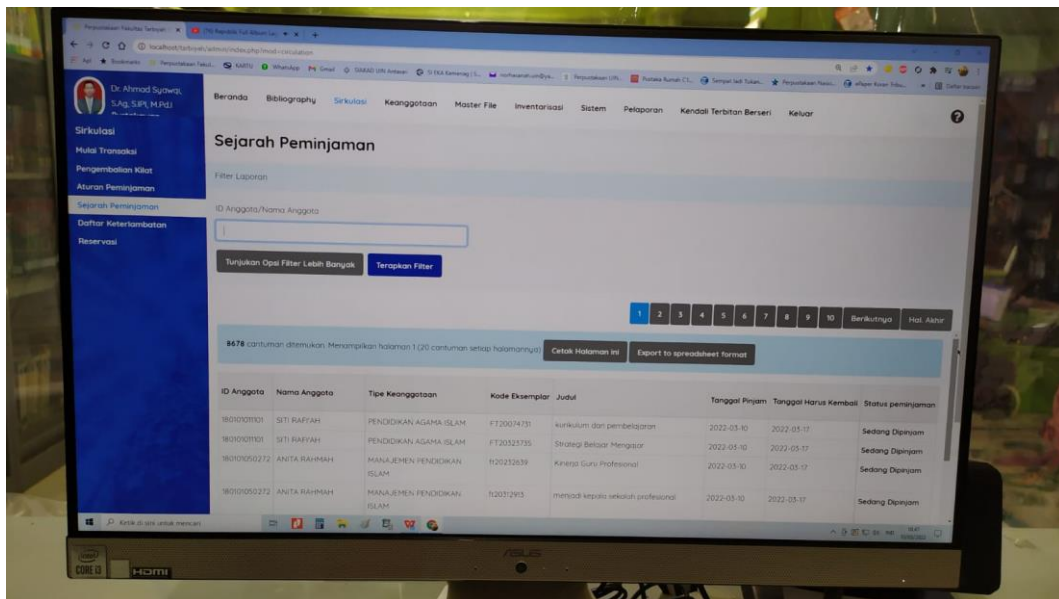
Gambar 8 Riwayat peminjaman
