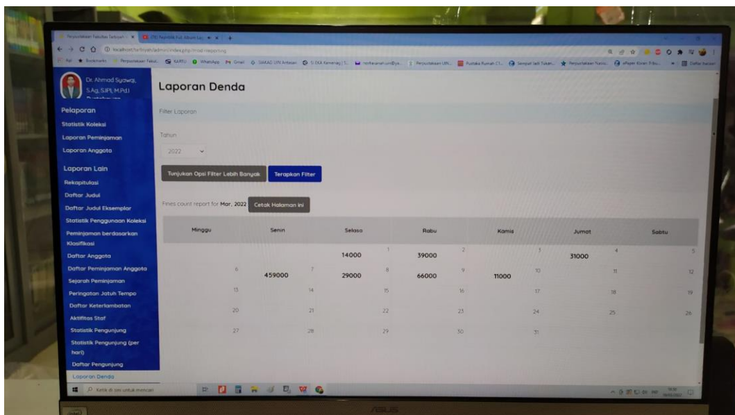
Gambar 11 Laporan denda
