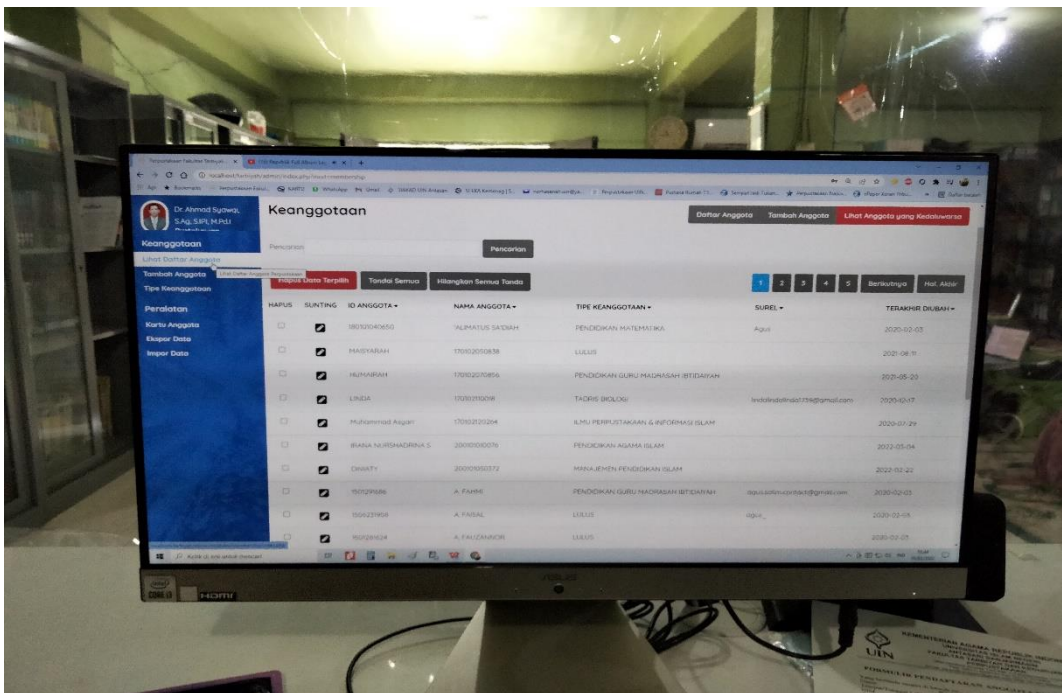
Gambar 5 Pendataan keanggotaan
