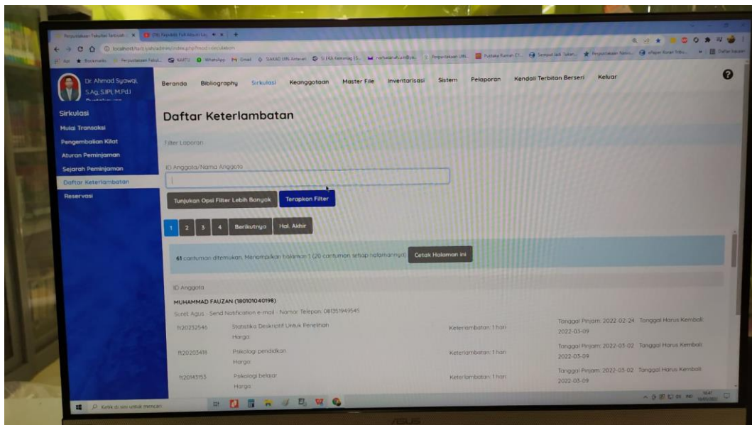
Gambar 10 Daftar keterlambatan
