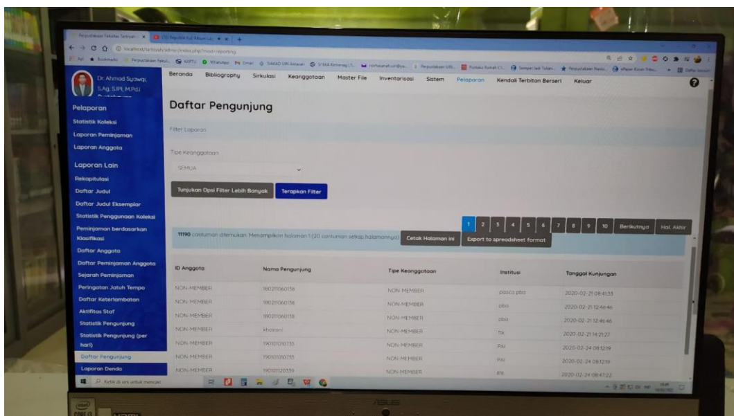
Gambar 9 Daftar pengunjung
