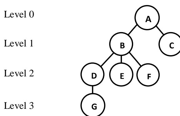
Gambar 4.1. Struktur Pohon
