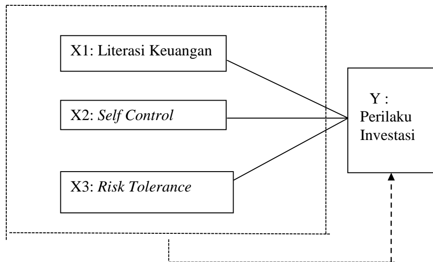
Gambar 1.1 Kerangka Berpikir
