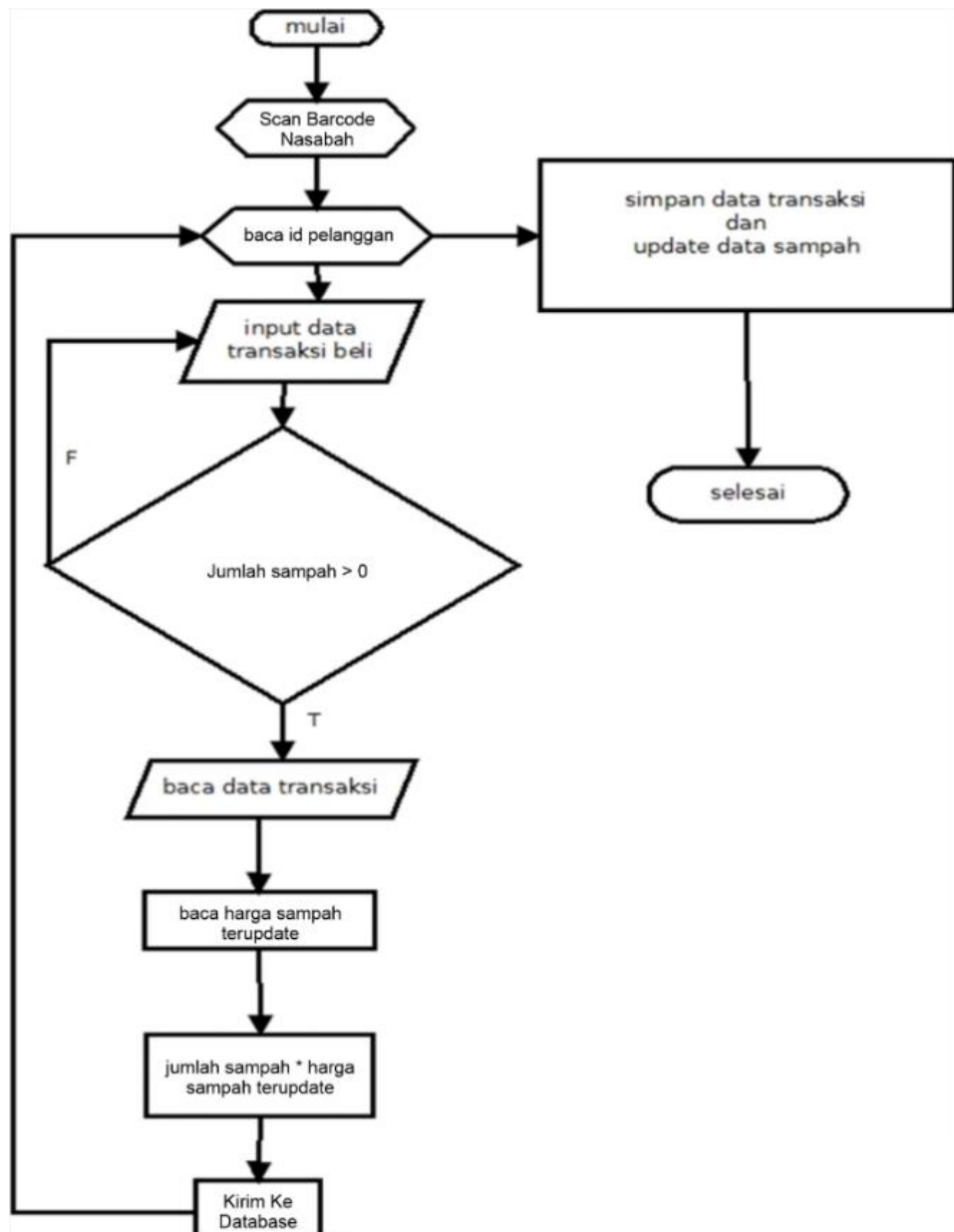
Gambar 4.22 Flowchart Transaksi Tambah
