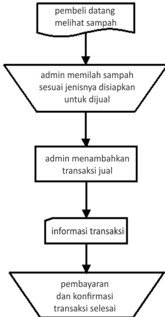
Gambar 4.21
