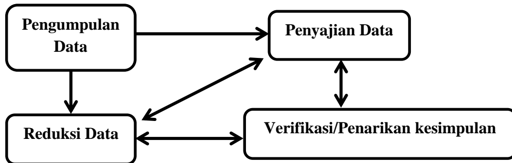
Gambar 3.1. Model Analisis Data Interaktif Miles dan Huberman
