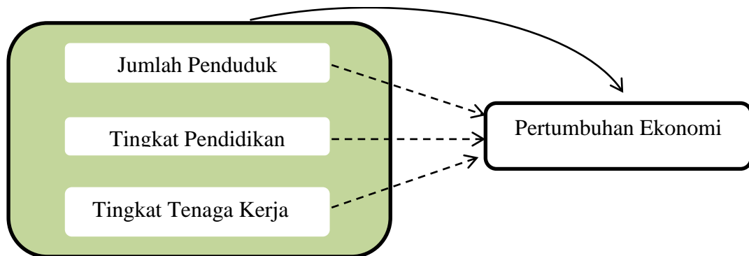
Gambar 1. 1 Kerangka Pemikiran
