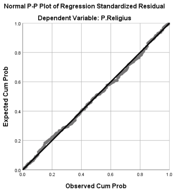
Grafik Uji Normalitas Data dengan P-P Plot Persamaan Pertama
