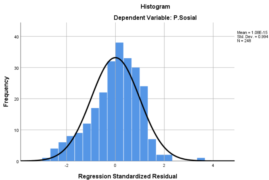
Grafik Uji Normalitas Data dengan Histogram Persamaan Kedua
