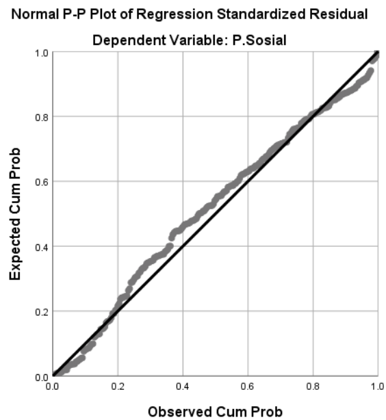
Uji Normalitas Data dengan P-P Plot Persamaan Kedu
