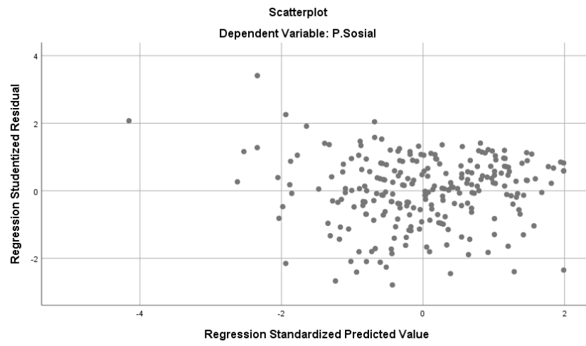
Grafik Hasil Scatterplot Persamaan Kedua
