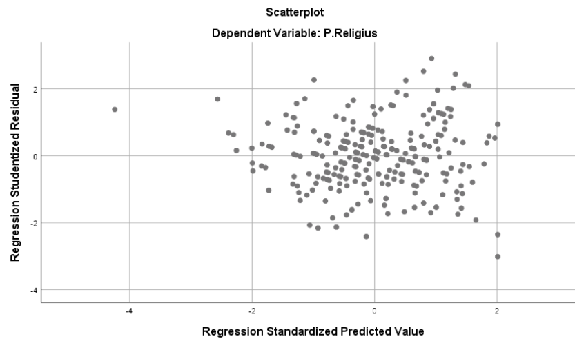
Grafik Hasil Scatterplot Persamaan Pertama
