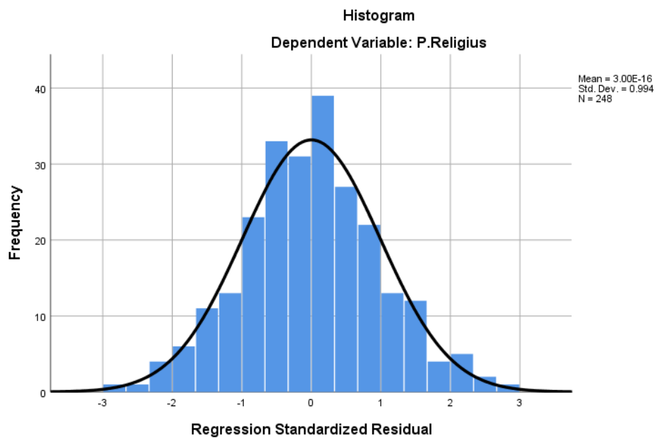
Grafik Uji Normalitas Data dengan Histogram Persamaan Pertama
