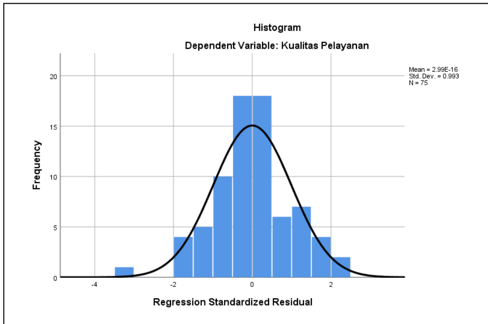
Gambar Uji Normalitas (Histogram)
