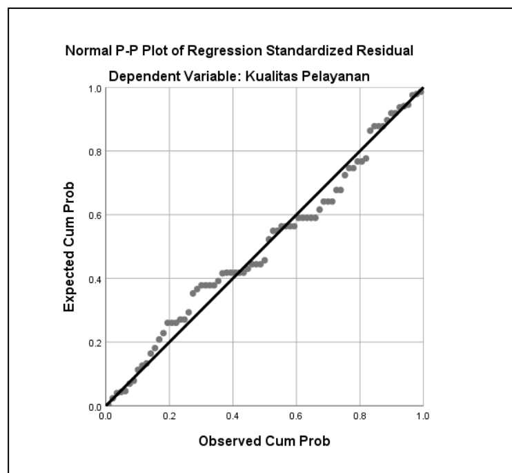
Gambar Uji Normalitas (Grafik P-Plot)
