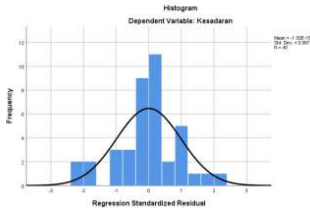
Gambar 4.1 Hasil Uji Normalitas Menggunakan Histogram
