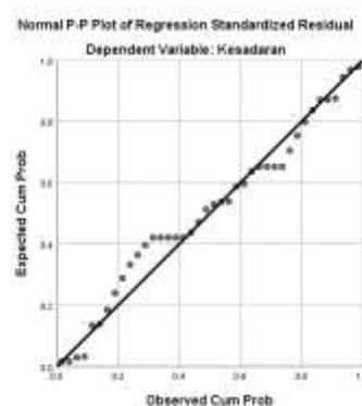
Gambar 4.2 Hasil Uji Normalitas P-P Plot
