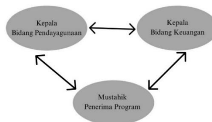
Gambar 3.1 Triangulasi Sumber
