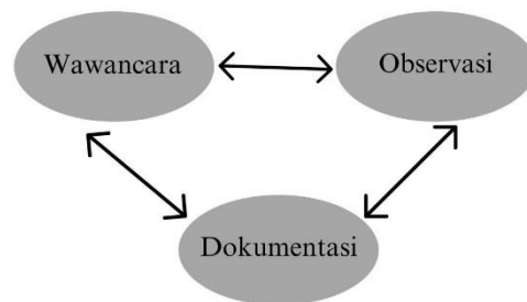
Gambar 3.2 Triangulasi Teknik
