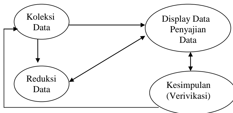
Bagan analisis Data Kualitatif menurut Miles dan Huberman
