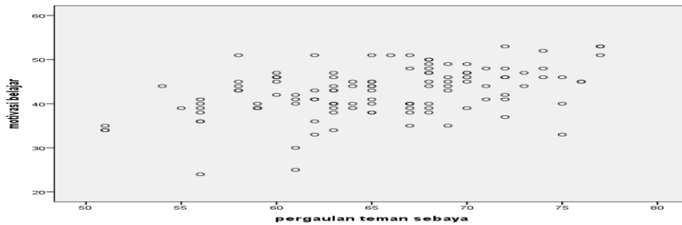
GRAFIK 4.3 Uji Linieritas
