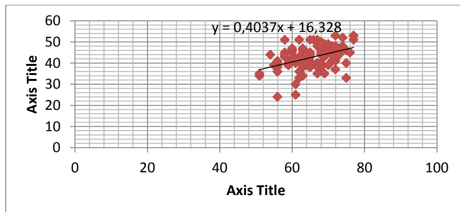
Grafik 4.4 Persamaan garis regresi
