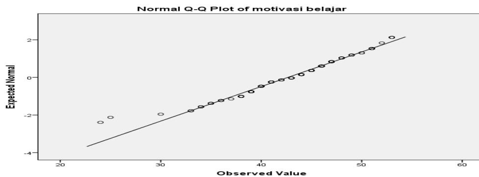
GRAFIK 4.2 Normal Q-Q Plot Motivasi belajar
